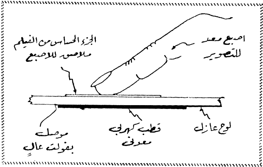
شكل ( ١١ ) يوضح بطريقة مبسطة كيفية الحصول على صورة لطرف اصبع بالتصوير الكيرلياني ، فتظهر له هالة على الفيلم الحساس نتيجة للتفريغ الكهربى ، وليس لطاقة روحية كما يزعم أنصار الروحانية .
